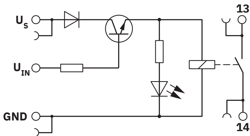
Schaltplan
