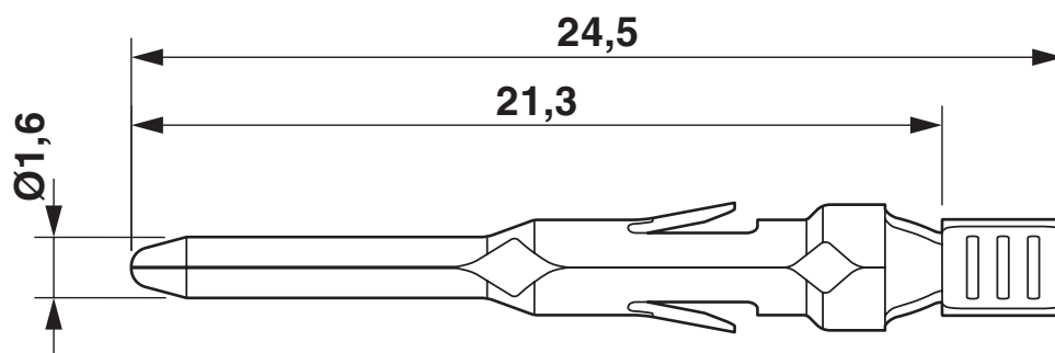
Dessin coté
