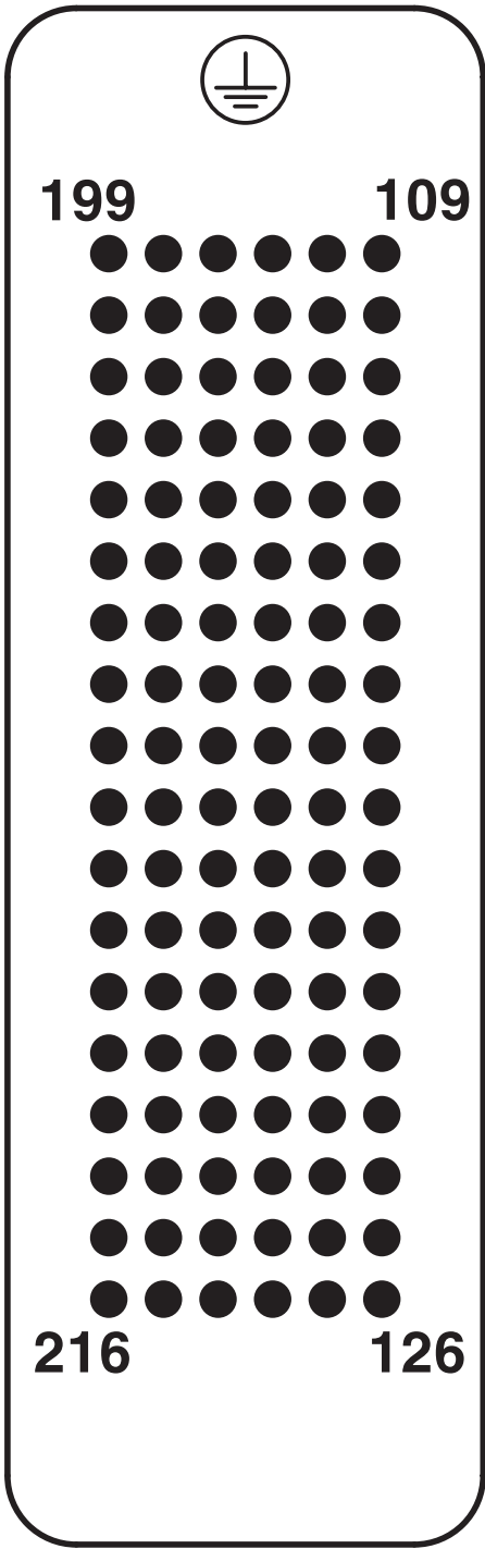
Plano esquemático
