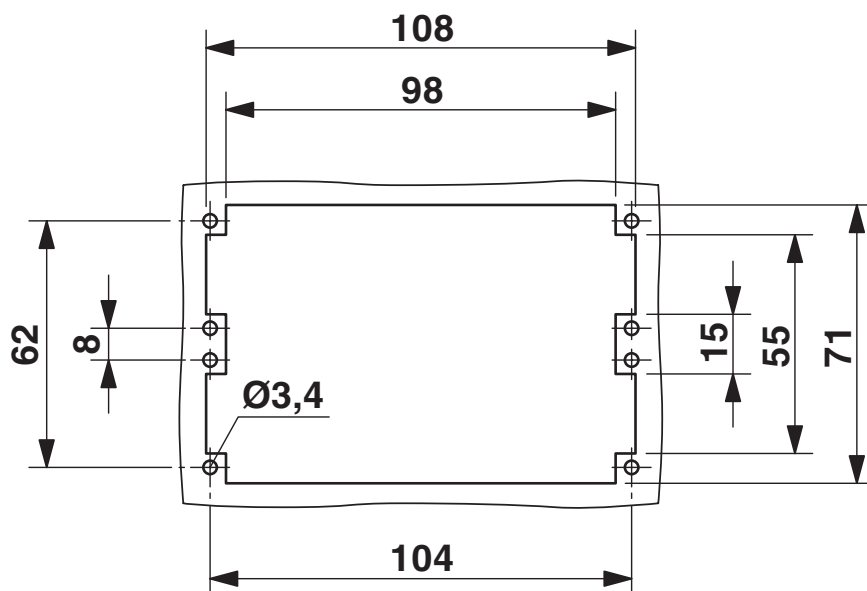
Dessin coté
