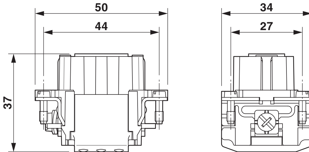
Maßzeichnung
