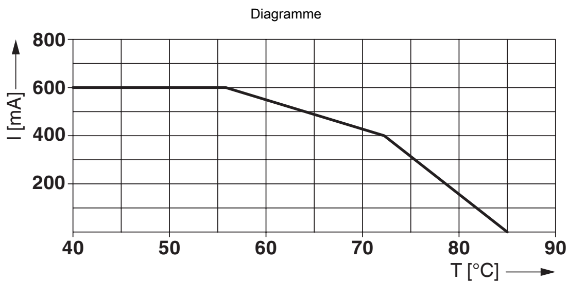
Courbe de derating à 30 V AC
