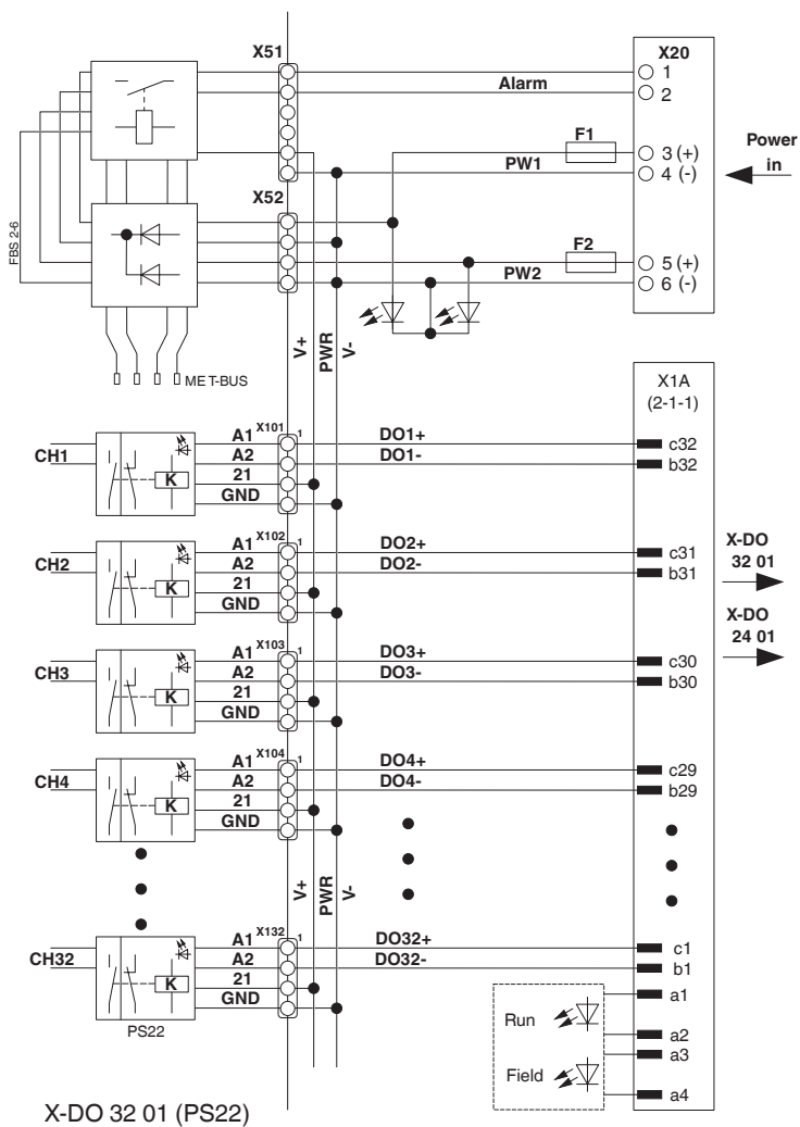
Blockschaltbild
