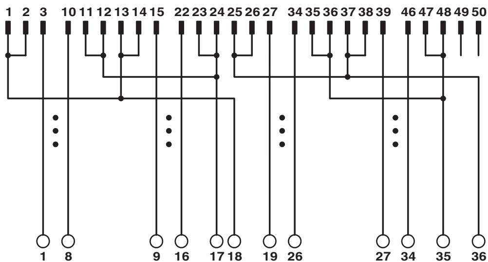
Schéma des connexions VIP-2/.../FLK50/AB-1756
