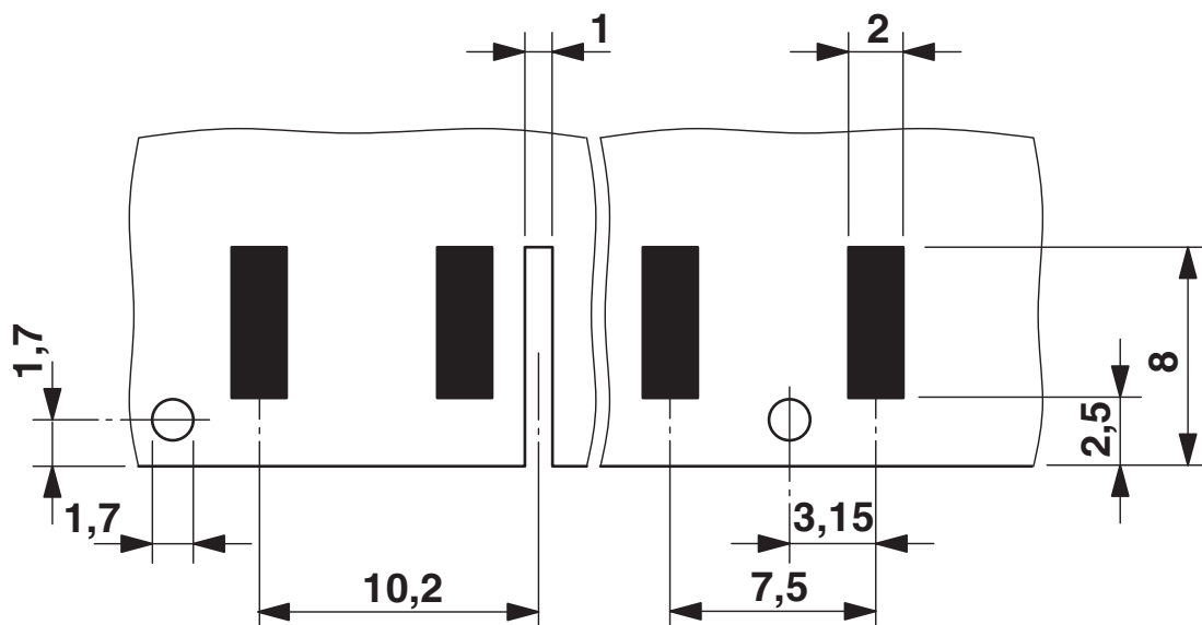
Esquema de taladros/geometría pads soldadura
