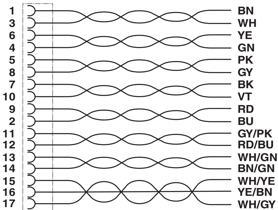
Schaltplan
