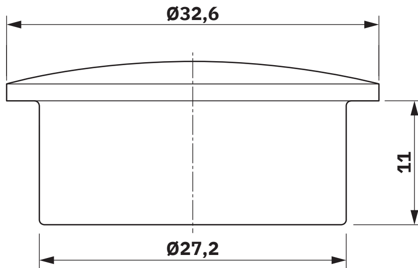
Maßzeichnung
