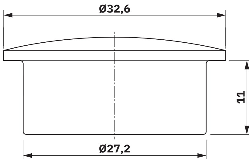
Dessin coté
