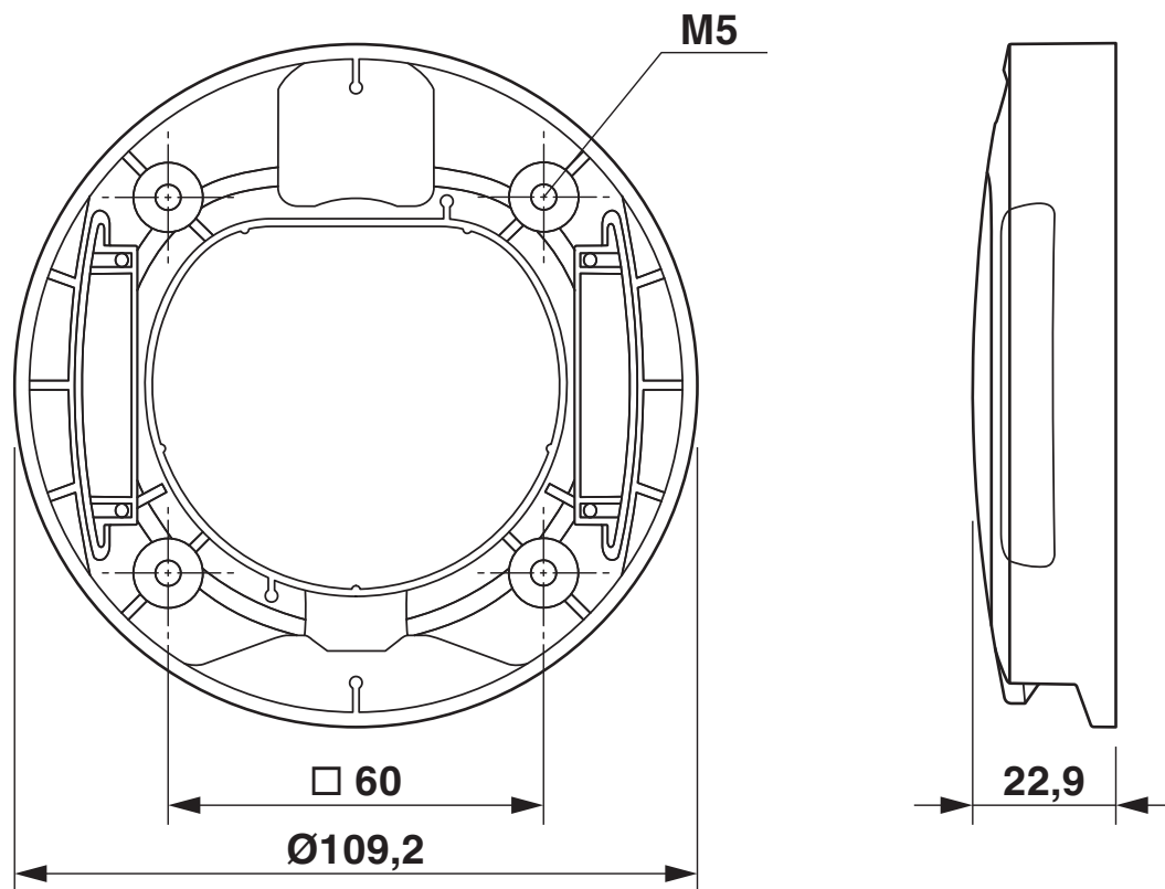
Dessin coté
