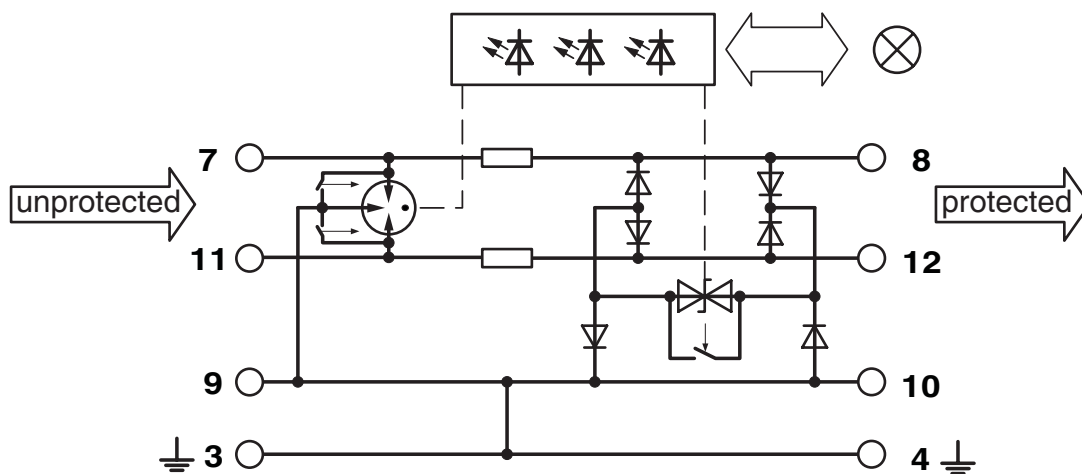
Diagrama eléctrico
