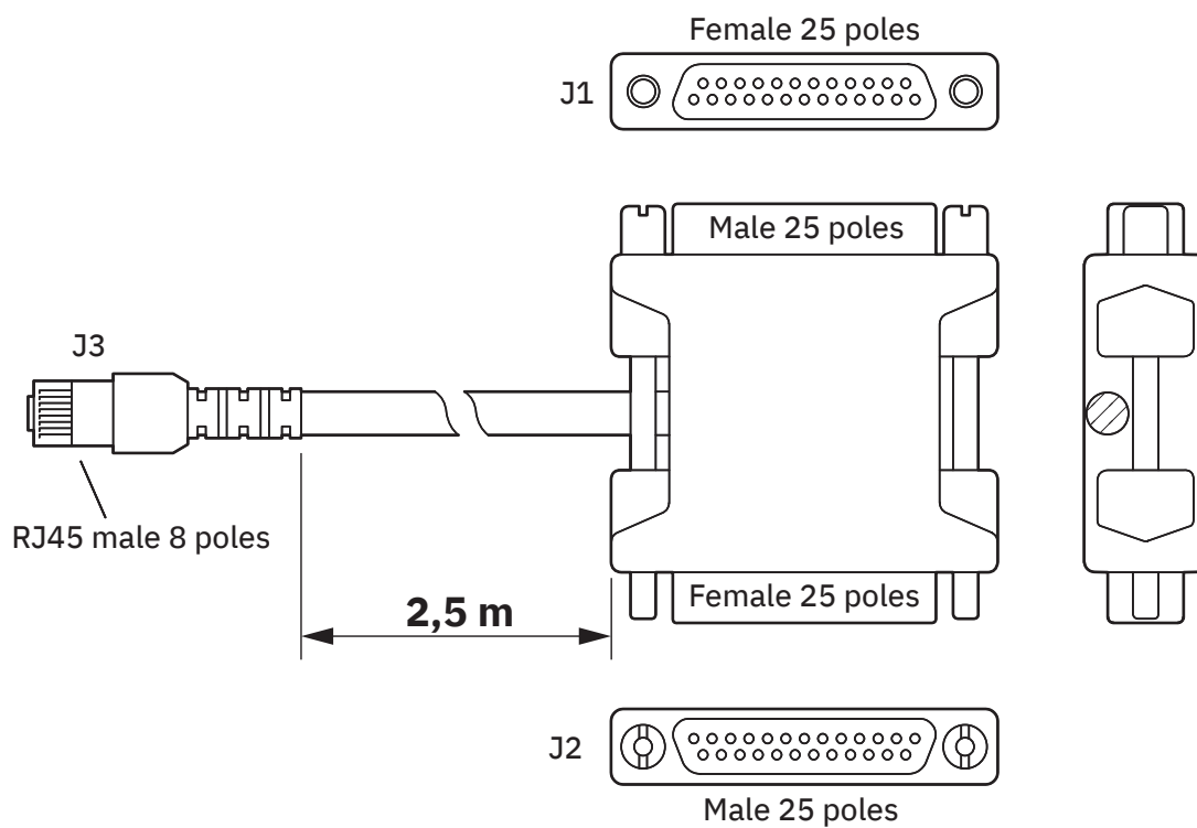
Plano esquemático
