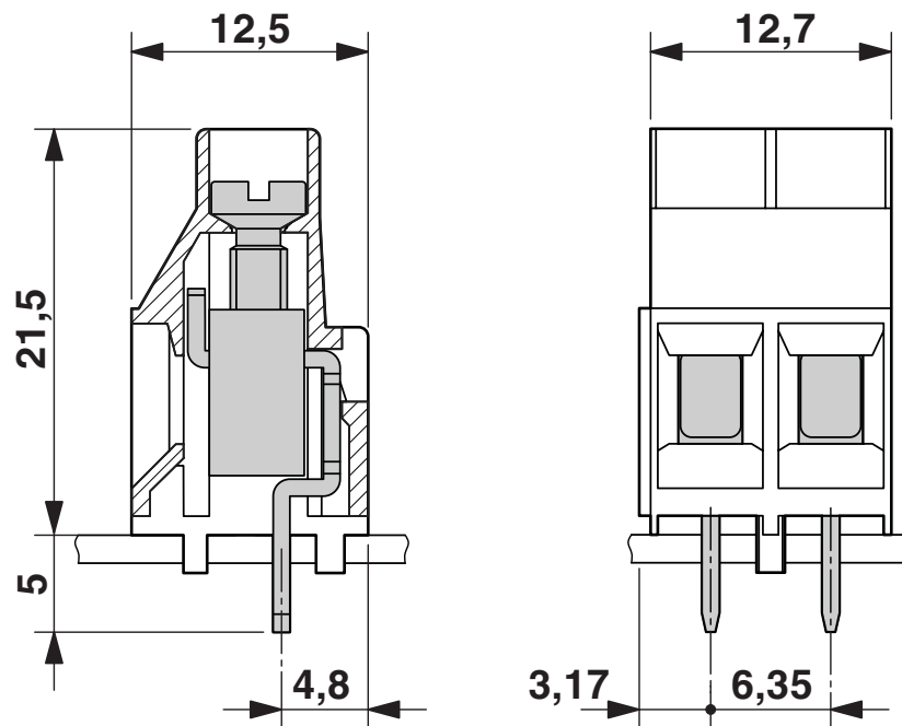
Maßzeichnung
