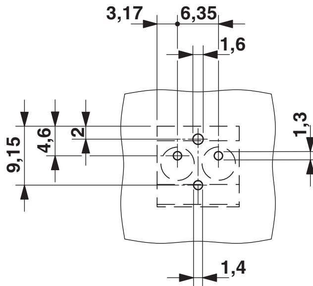
Bohrplan/Lötpadgeometrie
