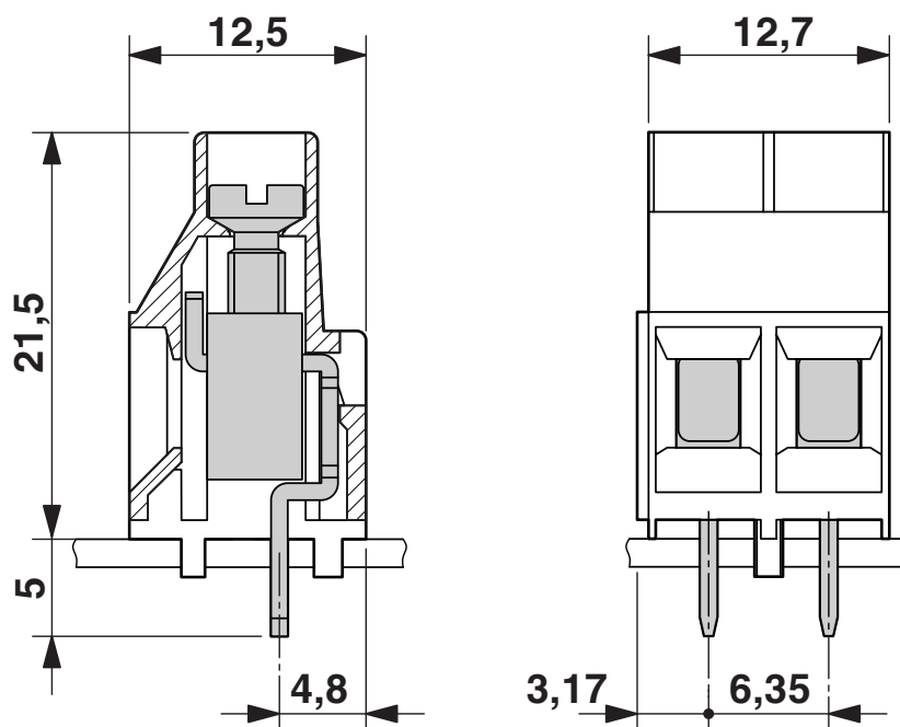
Dessin coté
