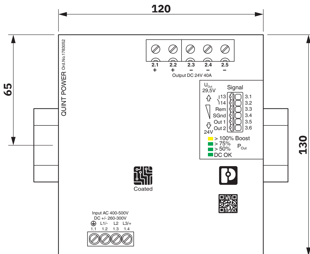
Abmessungen Vorderansicht (Maße in mm)
