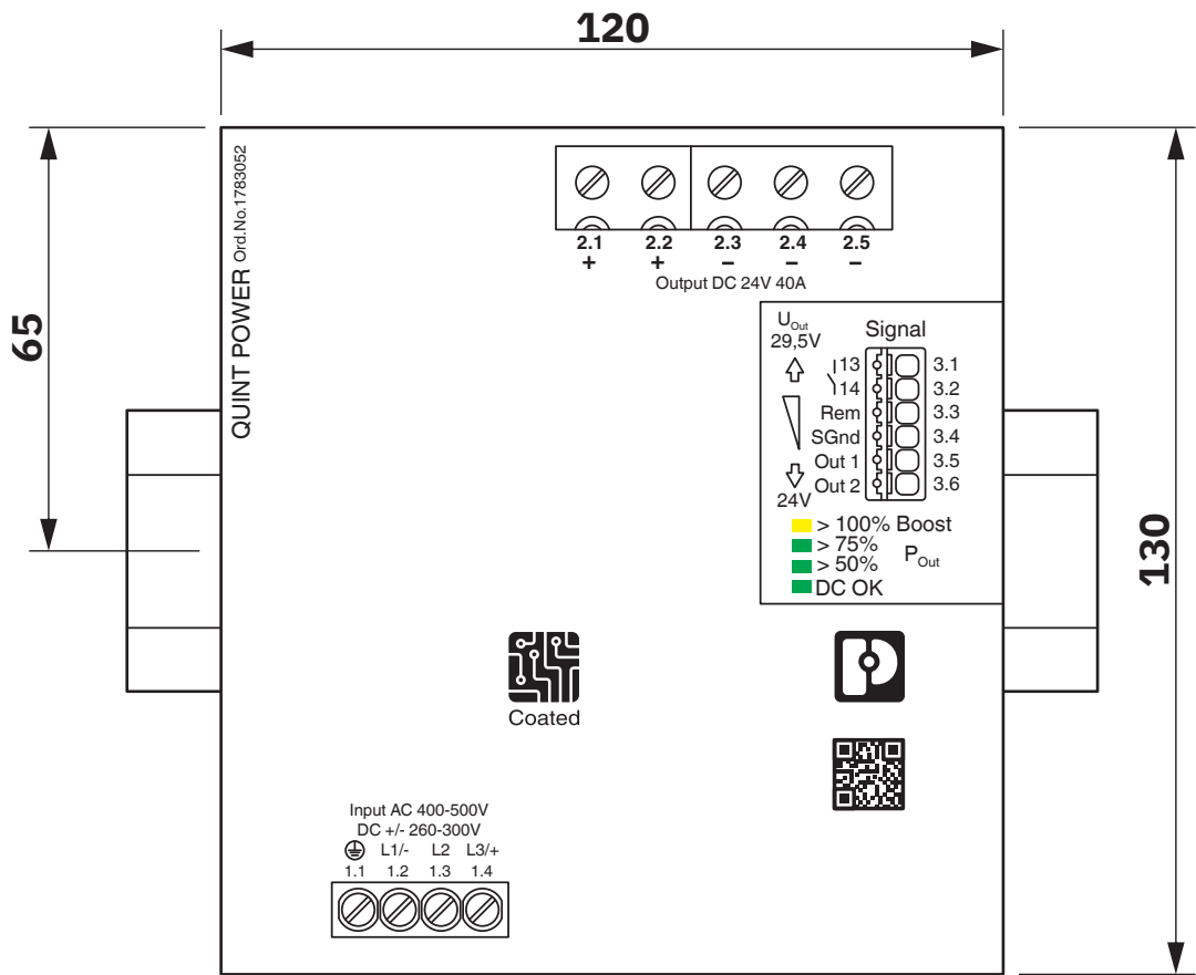
Dimensiones, vista frontal (en mm)
