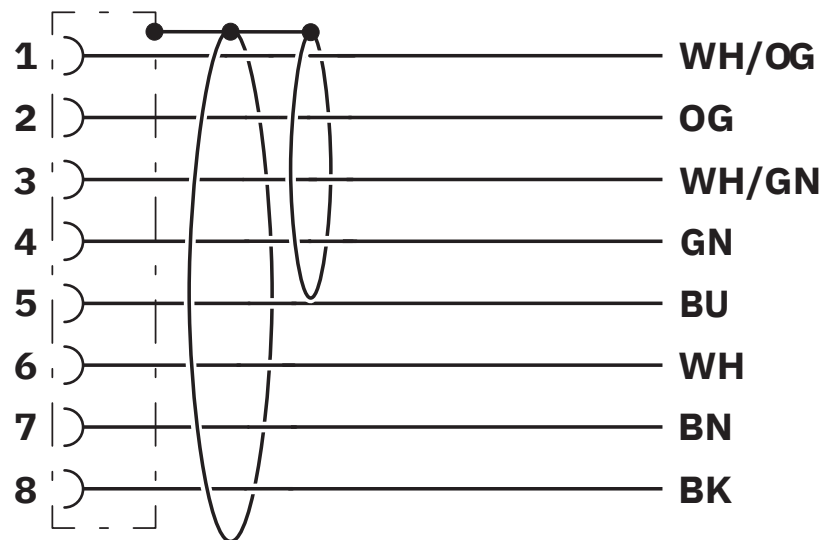
Schaltplan
