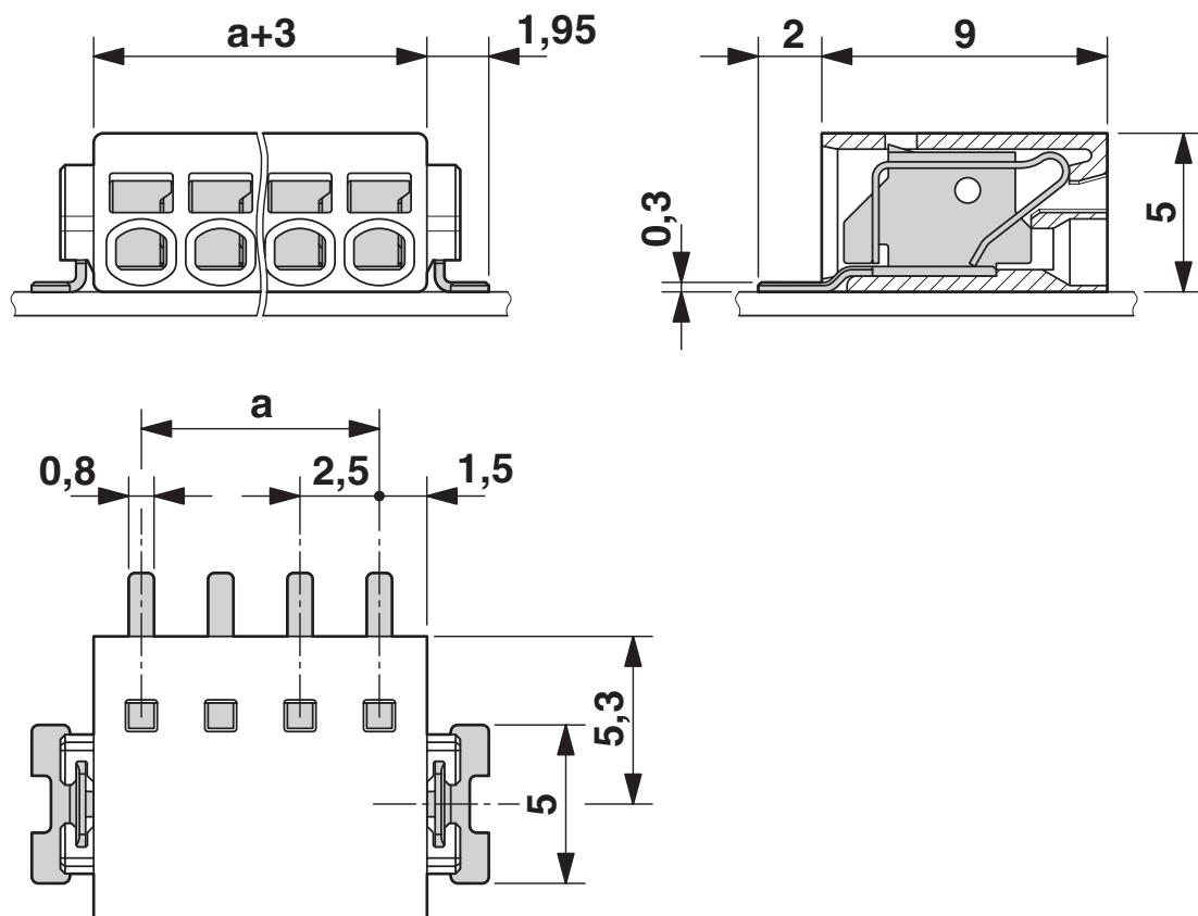
Maßzeichnung
