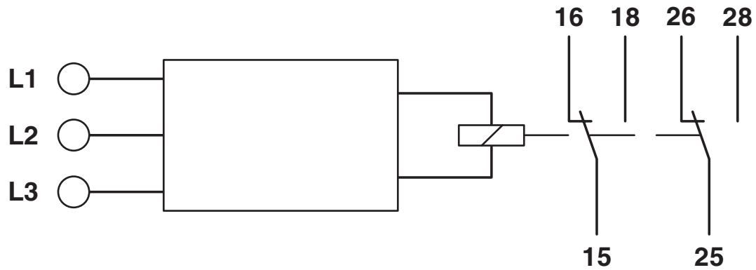
Schéma fonctionnel
