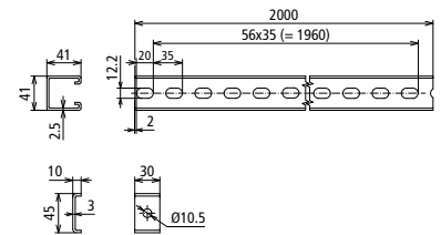
Maßbild MSC MDH V4A L2000 MZ V2A
