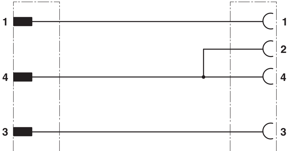
Schaltplan
