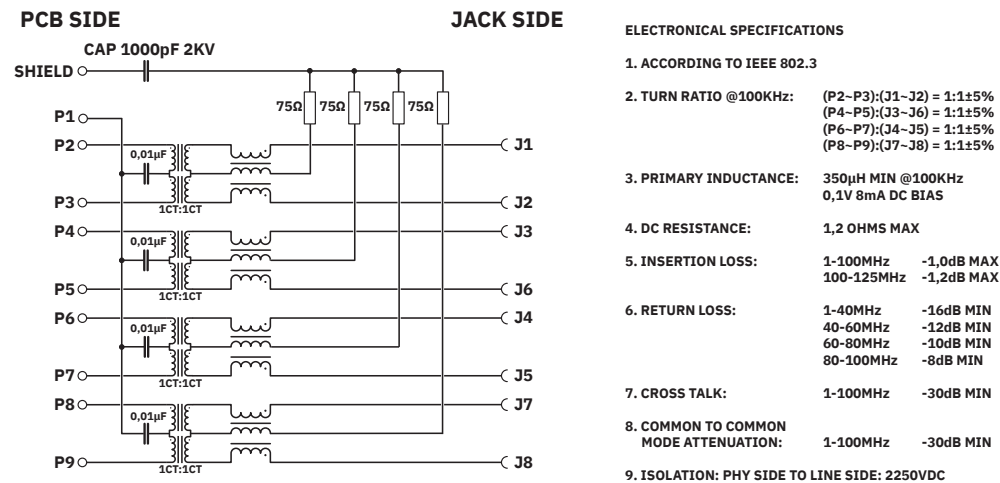
Diagrama eléctrico
