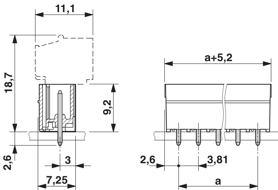
Dessin coté
