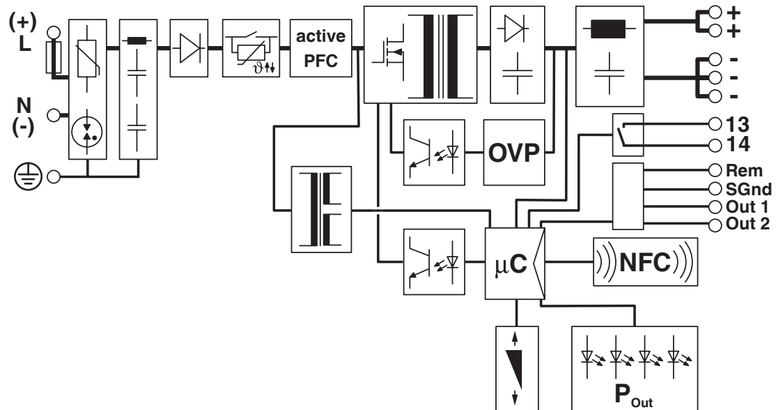
Blockschaltbild
