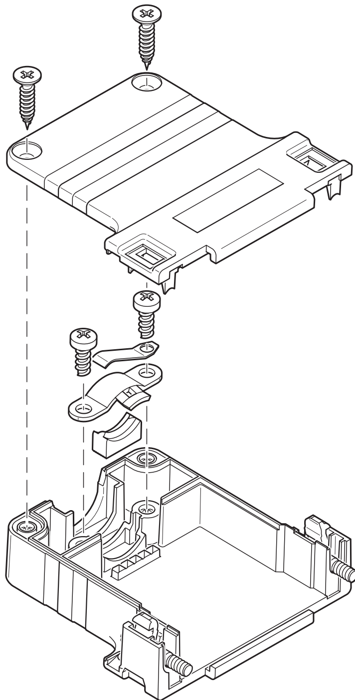
Plano esquemático
