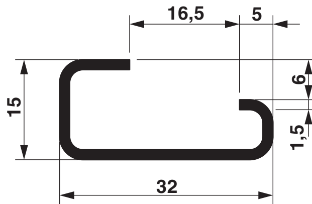
Maßzeichnung
