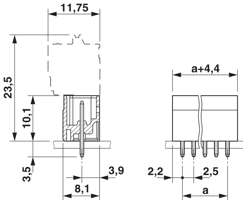
Maßzeichnung
