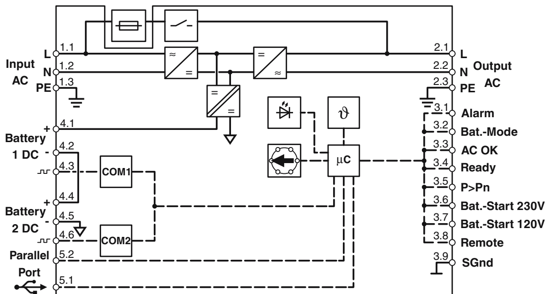
Schéma fonctionnel
