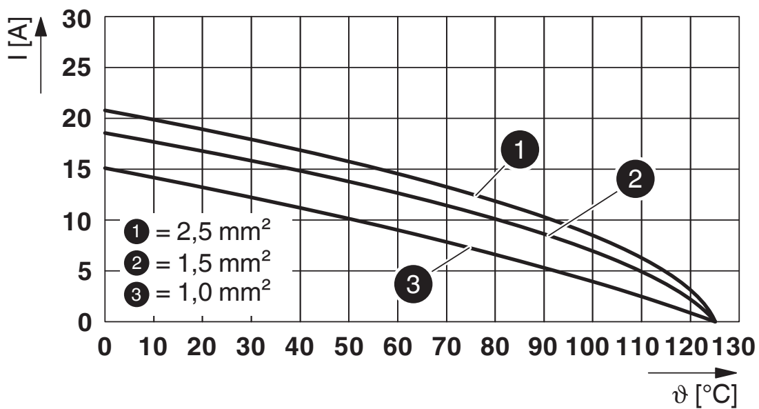
Diagrama derating de contactos mecanizados
