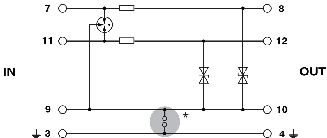
Diagrama eléctrico
