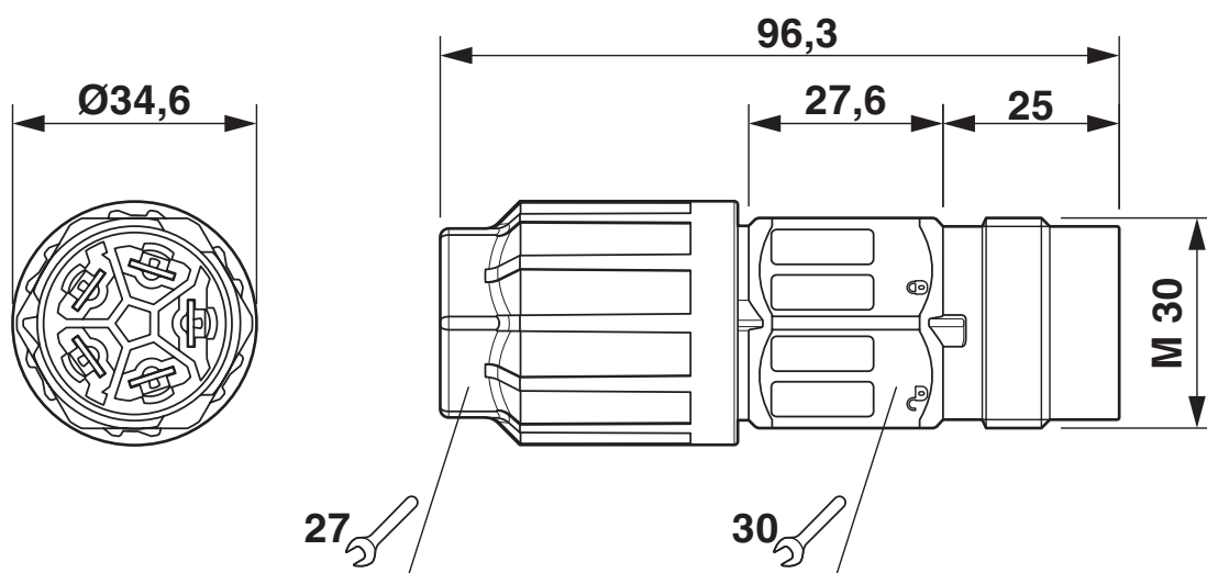
Dibujo acotado QPD C 5 x 2,5
