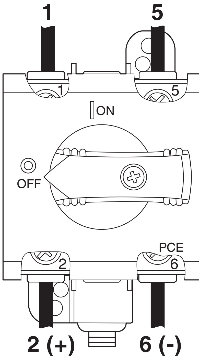
Dessin de la connexion
