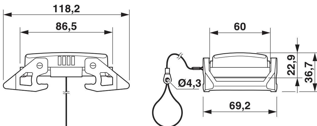
Dessin coté
