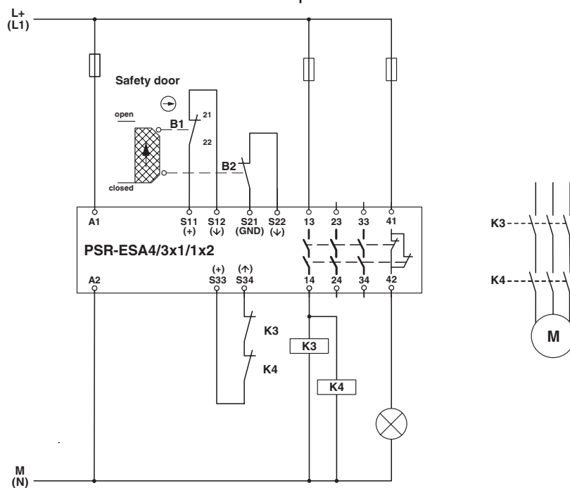
Schaltplan
