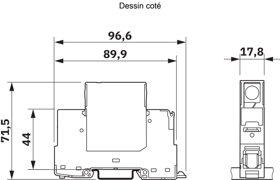
Dessin schématique
