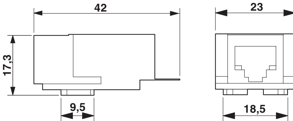
Maßzeichnung
