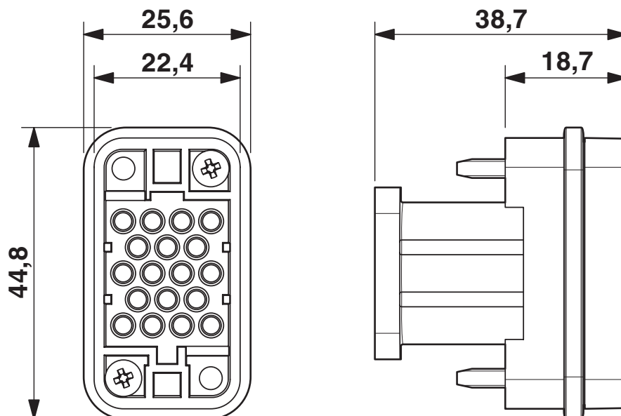
Esquema de dimensiones HC-COM-17-ESTC
