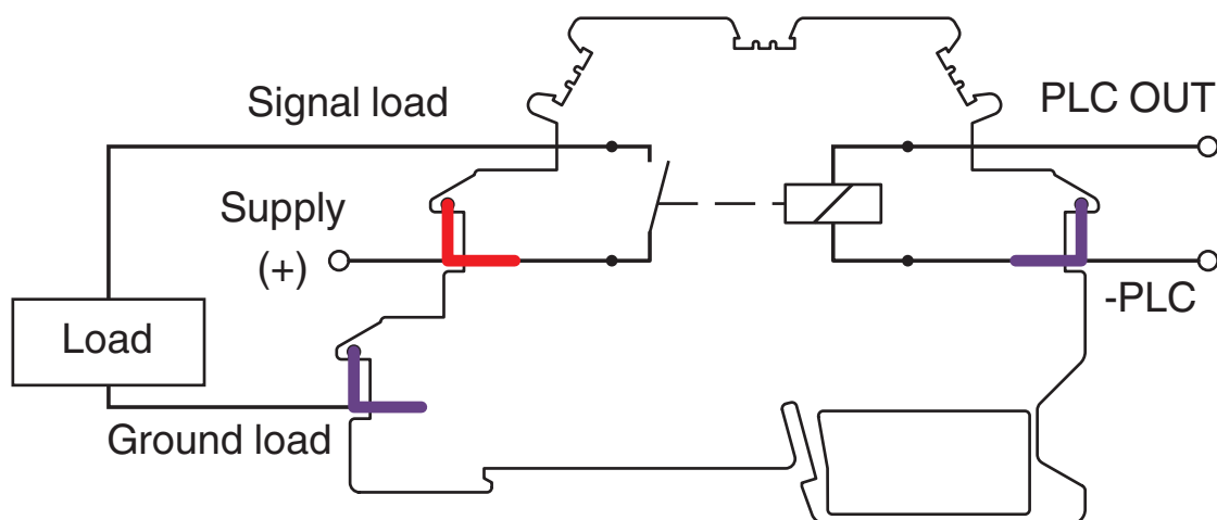
Anschlussbelegung DEK-REL-...AKT
