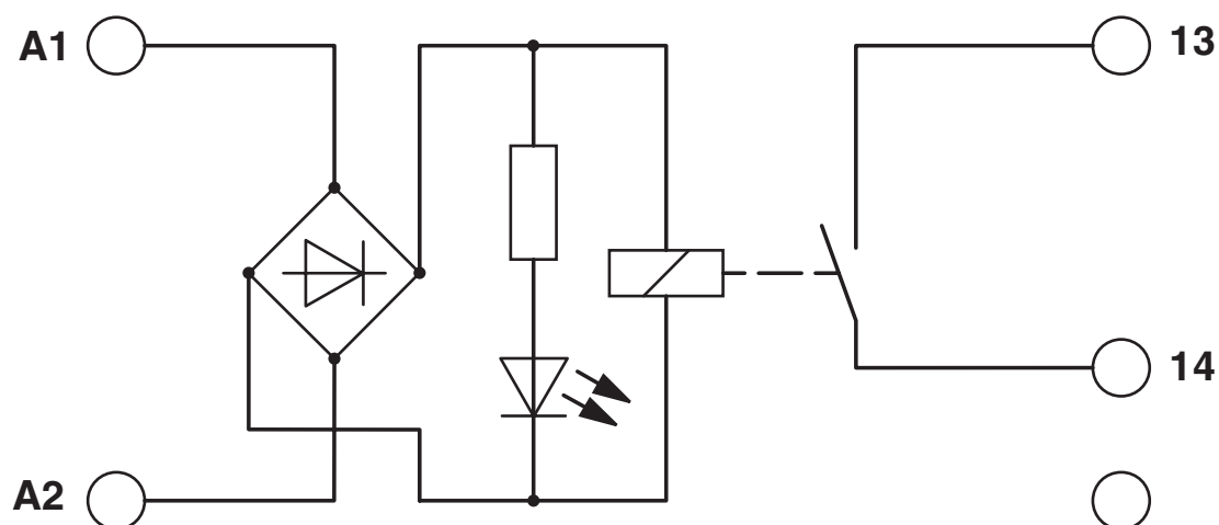
Schaltplan
