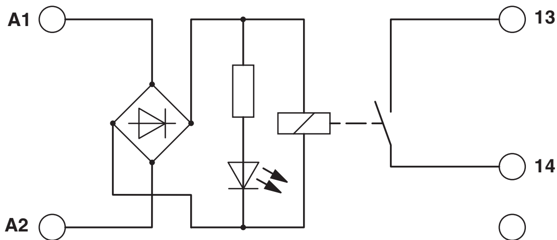
Diagrama eléctrico
