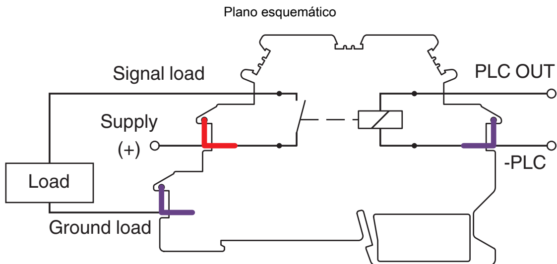
Diagrama eléctrico
