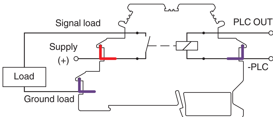
Plan des raccords DEK-REL-...AKT
