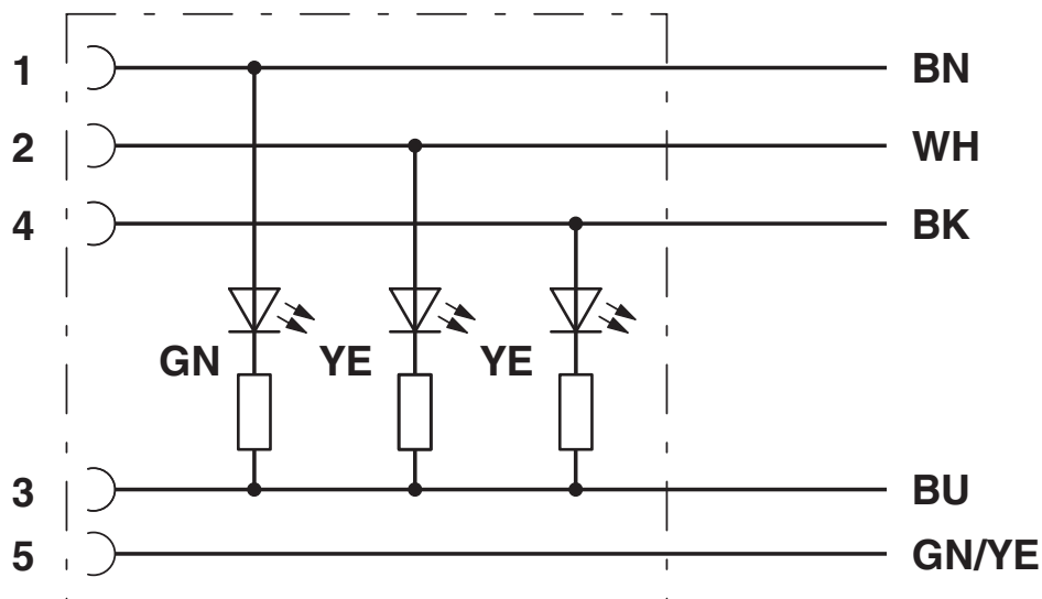
Diagrama eléctrico
