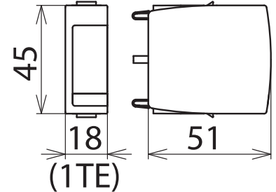
Maßbild DG MOD PV 600
