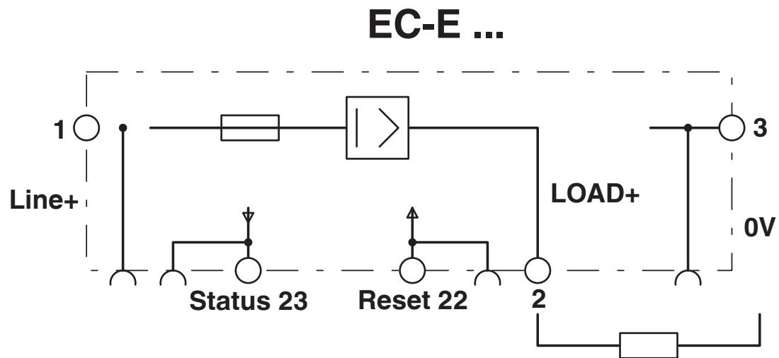
Diagrama eléctrico
