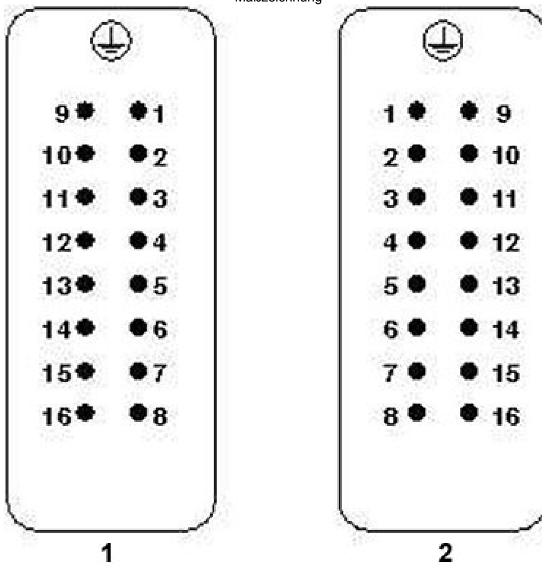
Maßzeichnung
