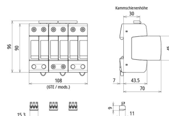
Dimensioni DG M DC ACI 1250 FM
