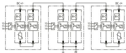
Schema di principio DG M DC ACI 1250 FM
