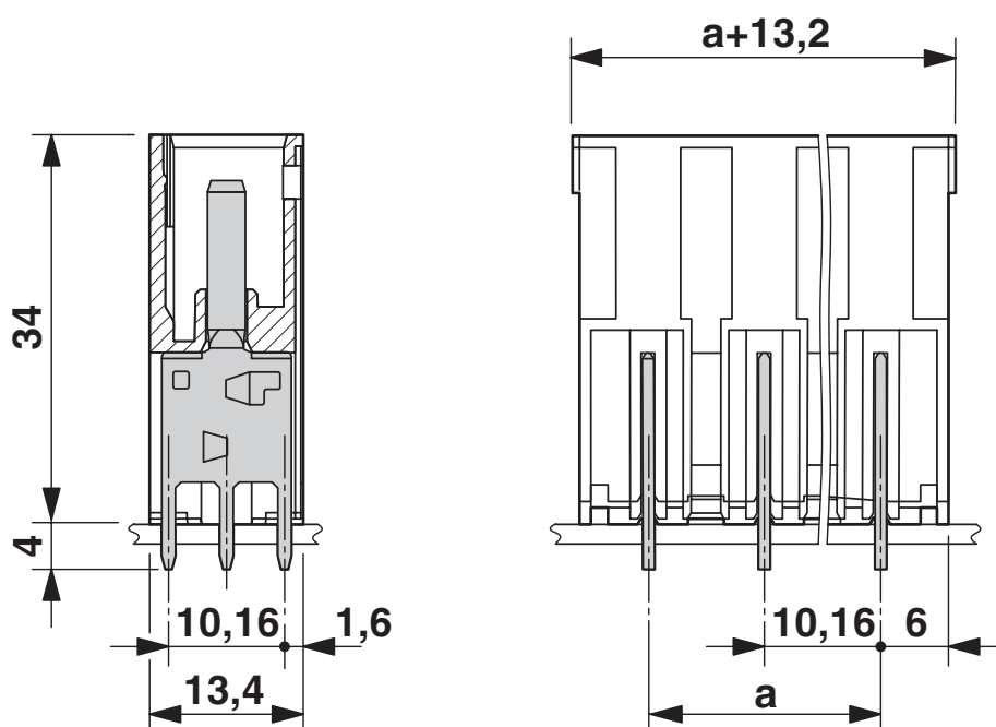
Dessin coté
