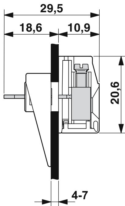
Dessin coté
